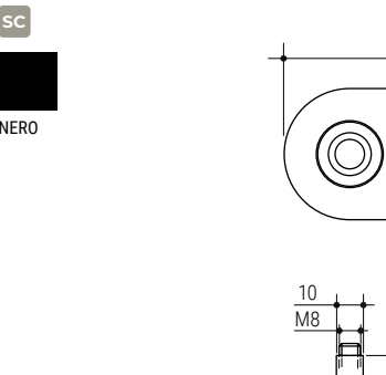
749 Piedino regolabile h 15 mm Regolable bearing h 15 mm 200 Pz
