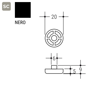
1845 Distanziale Ø 20 h 9 Spacer Ø 20 h 9 500 Pz
