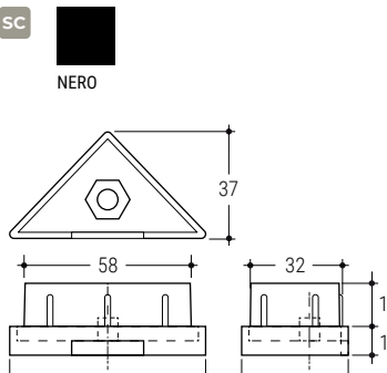
1743 Tappo terminale End cap 500 Pz
