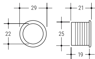
087B Senza fondo Without base Ø 29 h 19 VE VS VG GA SP
