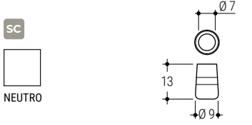
121 Q Paracolpo puntale Bumper tip
