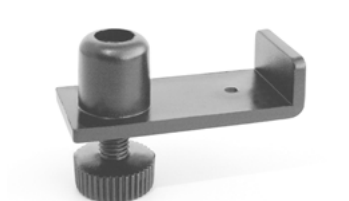
751 Piedino regolabile 60x25 h 8÷20 Regolable bearing 60x25 h 8÷20 500 Pz
