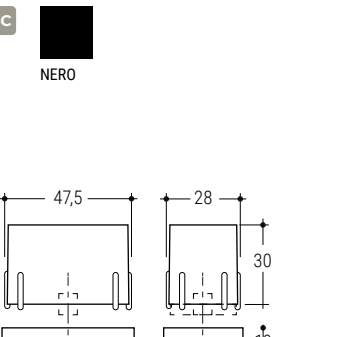
1610 P Tappo terminale End cap 500 Pz
