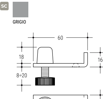
751 Piedino regolabile 60x25 h 8÷20 Regolable bearing 60x25 h 8÷20 500 Pz
