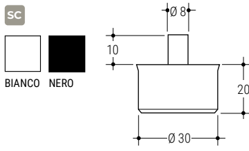
178 A Sottopiede di rialzo Lenghtening bearing
