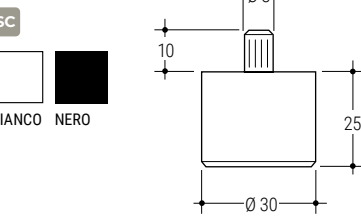
143 B Sottopiede di rialzo Lenghtening bearing
