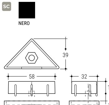
1744 Tappo terminale End cap 500 Pz
