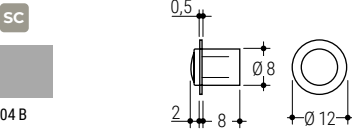
122 B Paracolpo ad incasso con battuta morbida Integrated bumper with soft edge
