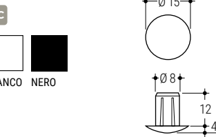
115 Piedino di rialzo Lenghtening foot
