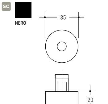
762 Piedino regolabile Ø 35 h 20 Regolable bearing Ø 35 h 20 500 Pz
