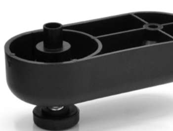
749 A Piedino regolabile h 27 mm Regolable bearing h 27 mm 120 Pz
