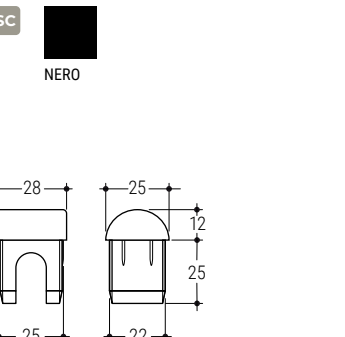
1849 Tappo terminale End cap 1000 Pz
