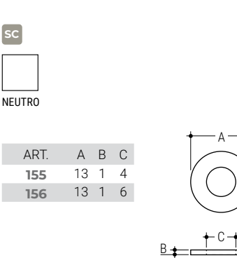
155-156 Rondelle distanziatrici Washer-spacers
