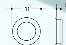
078B Ø 30,5 h 5 VE VS VG VM GA SP
