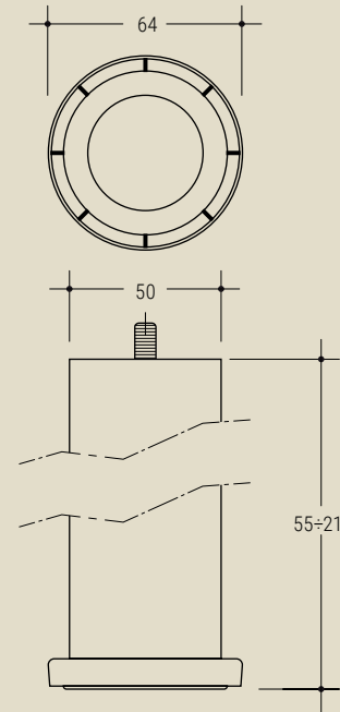
711B Ø 50/64 v. B2 h 55-65-75-85-95-105-115-125-135 145-155-165-175-185-195-205-215
